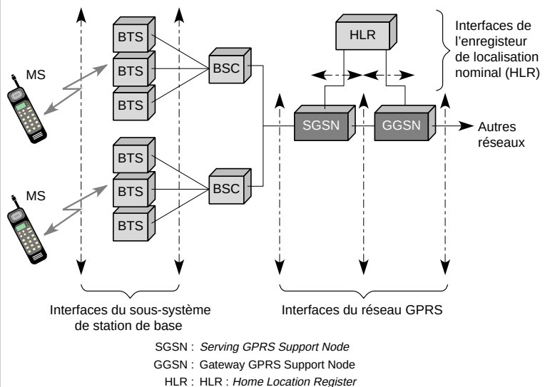
Figure 16-9. L'architecture du GPRS.
