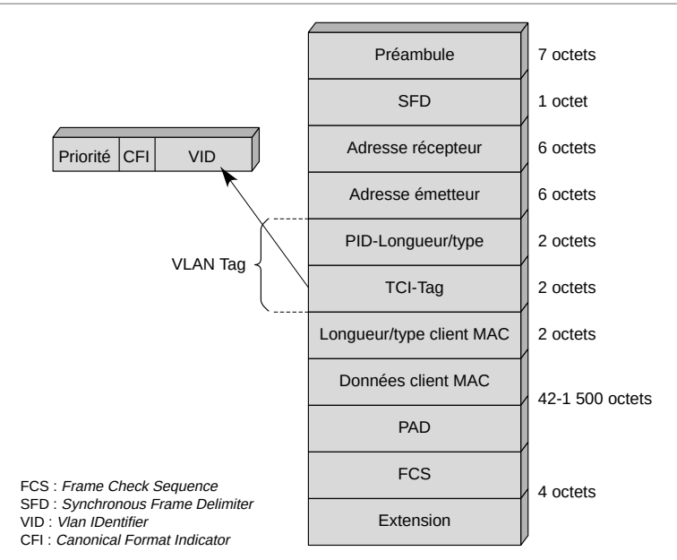
Figure 14-18. Le format de la trame Ethernet VLAN.
