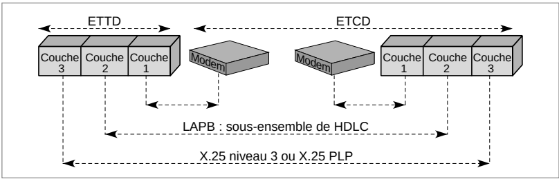
Figure 9-11. Les différents niveaux du protocole X.25.
