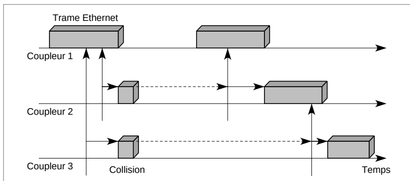
Figure 14-3. Le principe du CSMA/CD.
