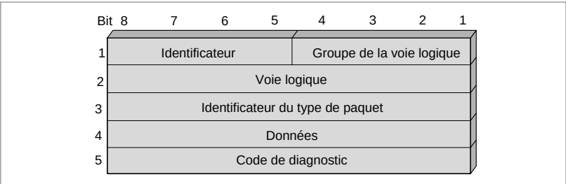
Figure 9-22. Le format des paquets de réinitialisation et de reprise.
