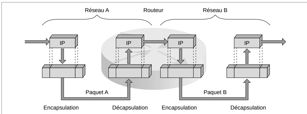
Figure 1-8. L'encapsulation-décapsulation d'un paquet IP.
