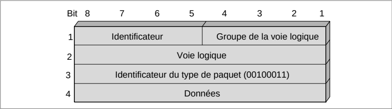
Figure 9-21. Les paquets d'interruption.
