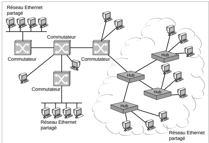
Figure 5-4. Une architecture complète de réseaux Ethernet.
