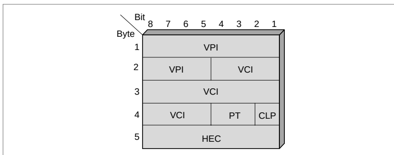
Figure 8-16. L'en-tête de la trame ATM sur l'interface NNI.
