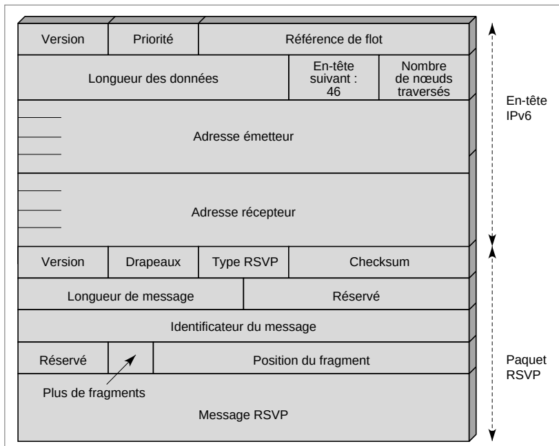
Figure 12-7. Le format du message RSVP.
